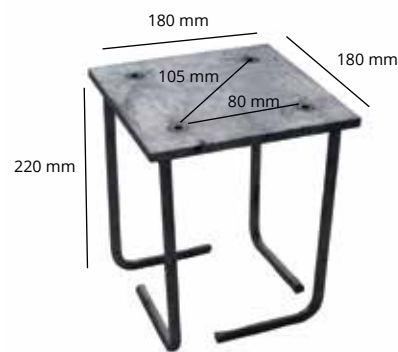
Grondanker
