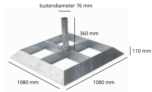
Tegelstandaard
