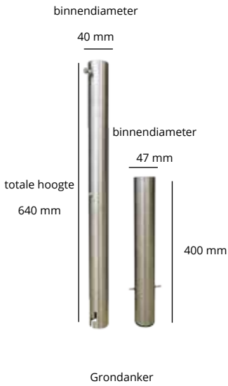
Grondanker
