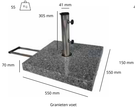
Granieten voet
