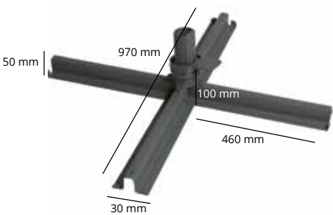
Kruisvoet
