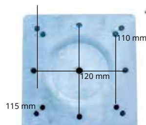
Ingraafvoet
