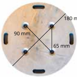
Adaptatieplaat
